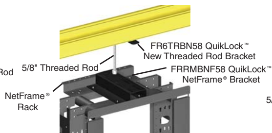
Mounting to Panduit® NetFrame® Rack
